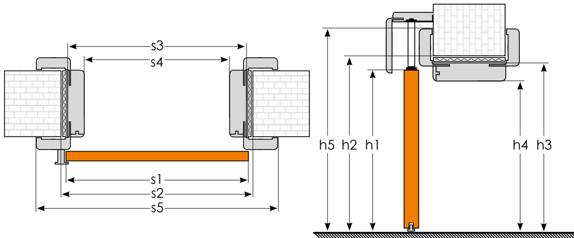
FAL ELŐTT FUTÓ TOLÓ RENDSZEREK TOK ÉS AJTÓLAP MÉRETEI (mm)
