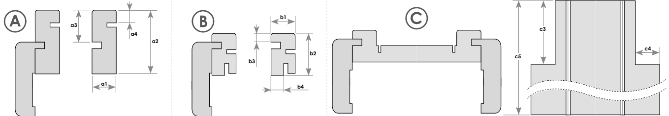
ÁBRA A FALBAN TOLÓ RENDSZER TOKSZÉLESÍTŐ ELEMEINEK ELHELYEKEDÉSÉRŐL
