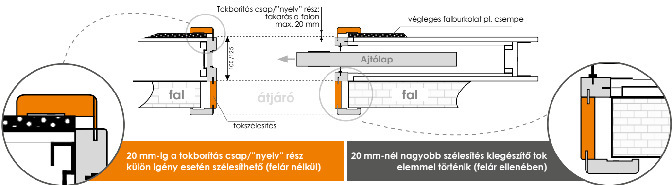
ÁBRA A FALBAN TOLÓ RENDSZER TOKSZÉLESÍTŐ ELEMEINEK ELHELYEKEDÉSÉRŐL
