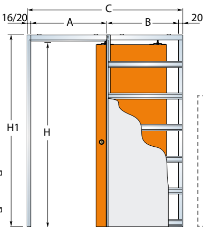
BEÉPÍTÉSI RAJZ AJTÓK TARTOZÉKOKHOZ A TOLÓ AJTÓKNÁL GIPSZKARTON FALHOZ
